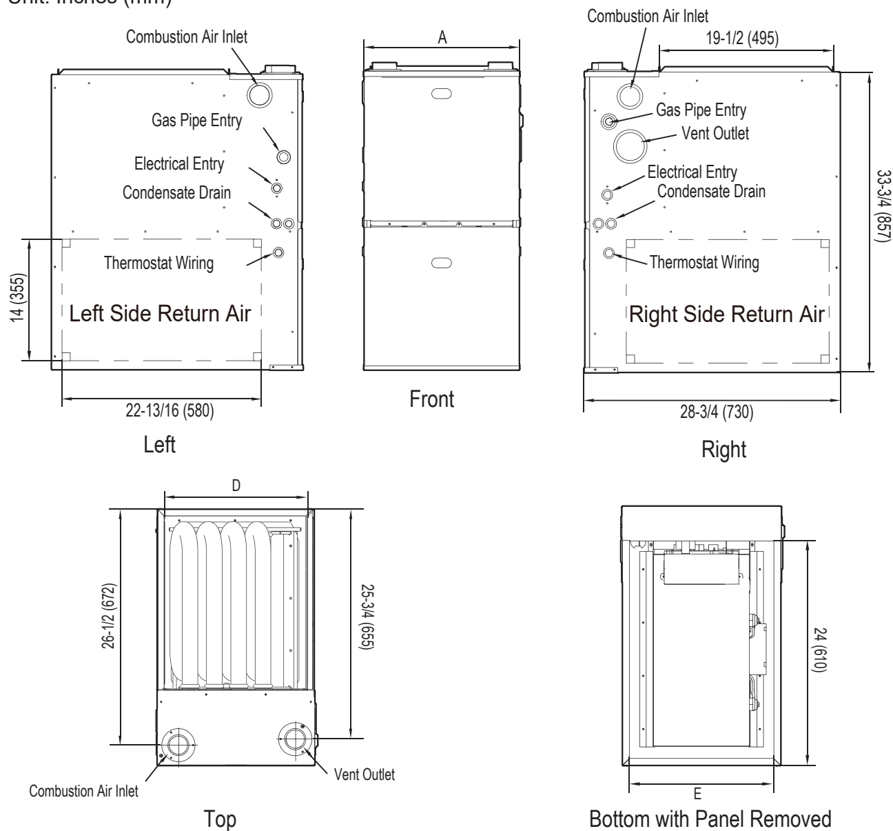
Figure 19: 96 AFUE Gas Furnace Unit Dimensions.
