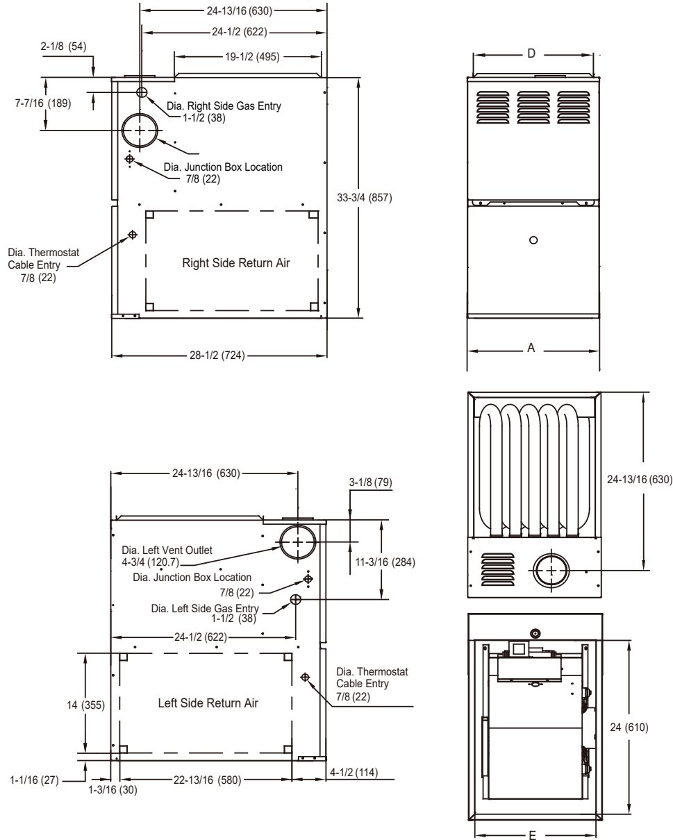
Figure 18: 80 AFUE Gas Furnace Unit Dimensions.
