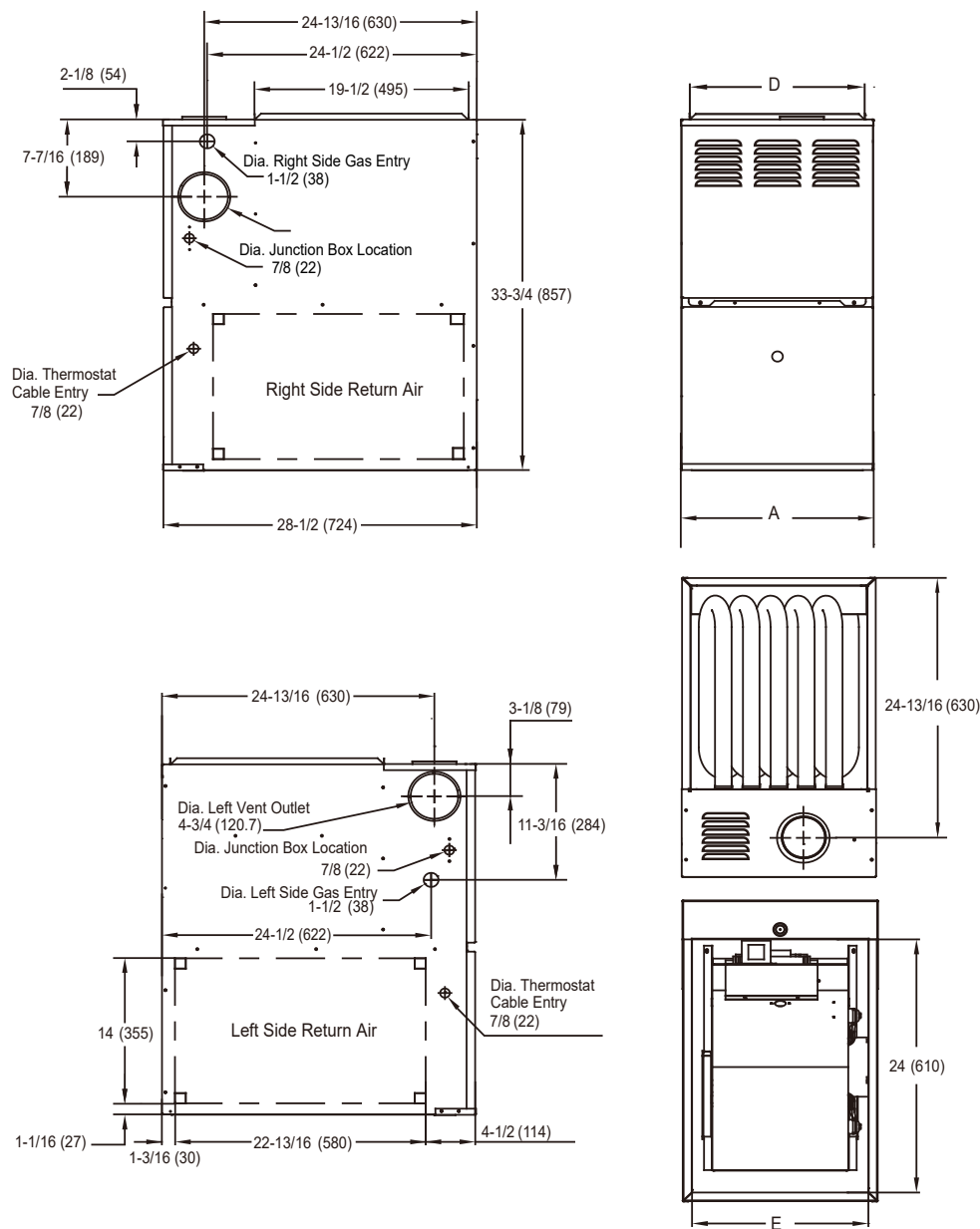
Figure 15: 80 AFUE Gas Furnace Unit Dimensions.
