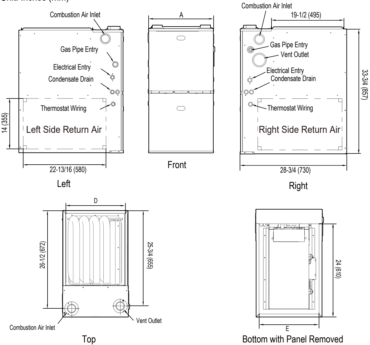
Figure 20: 96 AFUE Gas Furnace Unit Dimensions.
