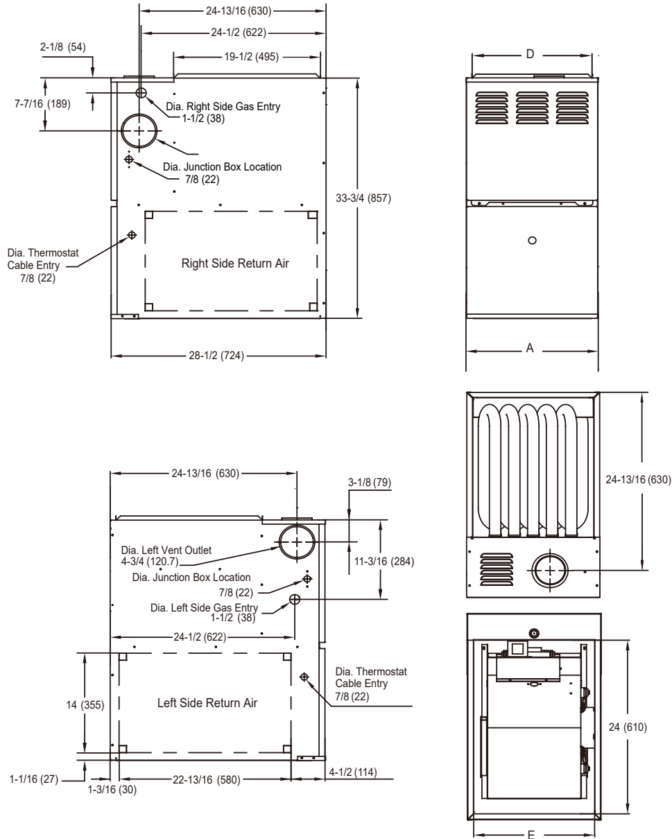
Figure 19: 80 AFUE Gas Furnace Unit Dimensions.
